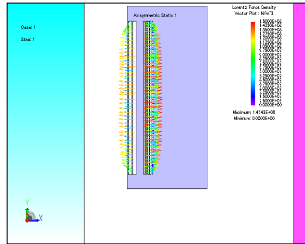
شکل (۸): مؤلفه های نیروی اتصال کوتاه وارد بر سیم پیچ
