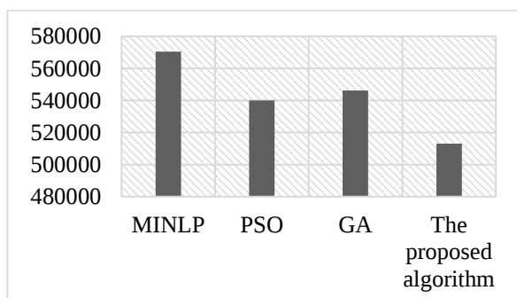
شکل (۷): نمودار ستونی مقایسه نتایج خروجی الگوریتم‌های GA^{[۱۶]} ، MINLP^{[۱۲]} ، PSO^{[۱۵]} (نمودار بر اساس خروجی تابع هدف (هزینه) می باشد)
