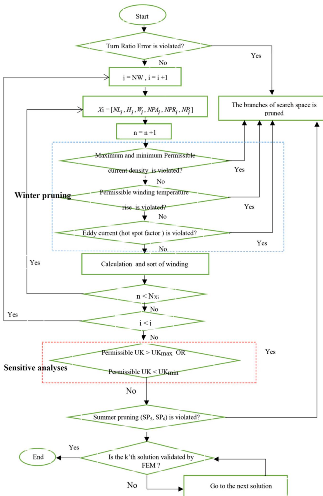
شکل (۱): فلوچارت الگوریتم ارائه شده [۱۱]
