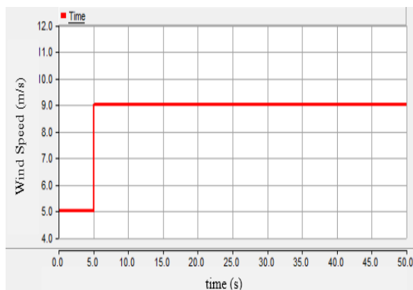
شکل (۷): منحنی تغییرات سرعت باد اعمالی به توربین‌های
