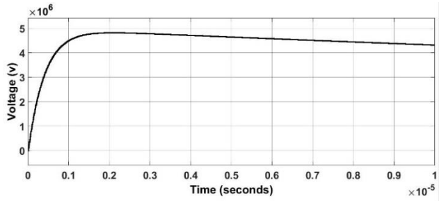
شکل ۳: موج ولتاژ ضربه ای استاندارد شبیه سازی شده با پیک ولتاژی 5MV
