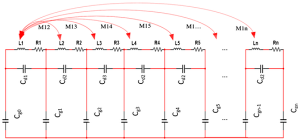
شکل ۴: ساختار سیم پیچ مدل دقیق یک ترانسفورماتور قدرت [۲۳]
