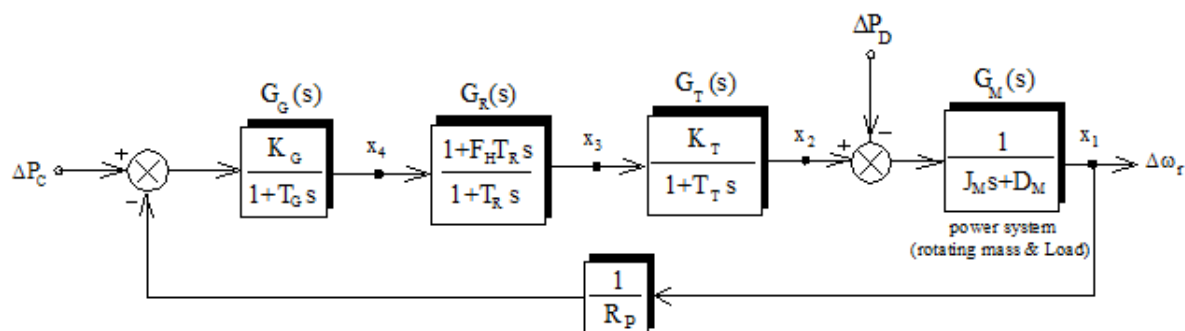
شکل (۱): بلوک دیاگرام واحد تولید با توربین بخار مجهز به باز حرارت ده
