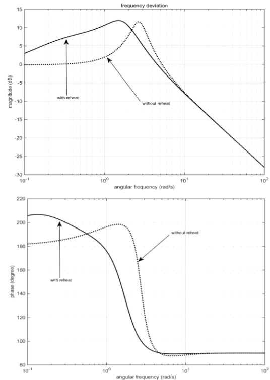
شکل (۴): پاسخ فرکانسی تابع انتقال تغییرات فرکانس به تغییرات ورودی بار
