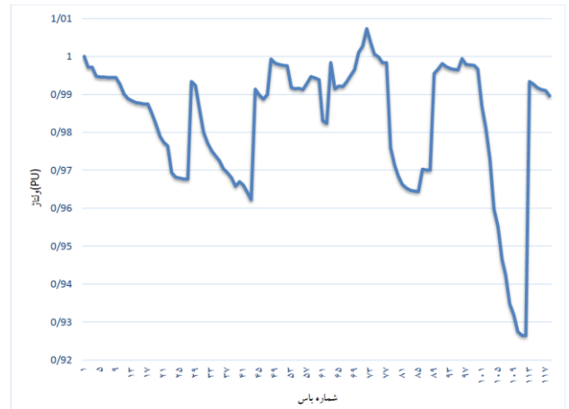
شکل (۱۵): پروفیل ولتاژ شبکه توزیع با جایابی سه DG و چهار خازن با عدم حذف خطوط ۴۳، ۶۵ و ۸۸
