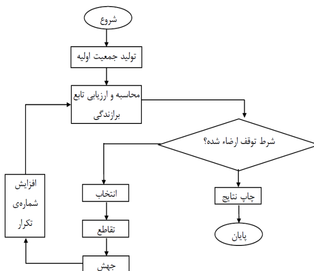
شکل (۲): فلوجارت اجرای الگوریتم ژنتیک
