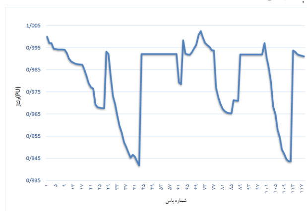
شکل (۱۳): پروفیل ولتاژ شبکه توزیع با جایابی یک DG و چهار خازن با حذف خطوط ۴۳، ۶۵ و ۸۸
