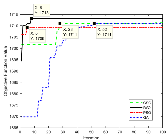
شکل(۲): نمودار همگرایی روش‌های مختلف بهینه‌سازی در سیستم ۱۴ باس IEEE برای حالت مبنا
