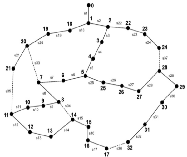
شکل ۲. دیگرام تک‌خطی شبکه آزمون ۳۲ شینه
