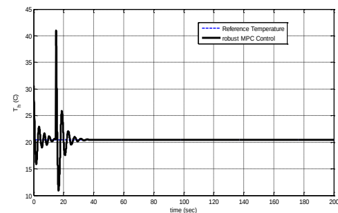
شکل (۱۲): متغیر خروجی دمای سطح منبع گرمایی با اعمال کنترل‌کننده‌ی ترکیبی پیش‌بین مقاوم (حالت دوم)
