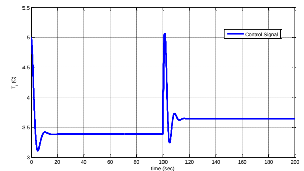
شکل (۱۹): سیگنال کنترل پیش‌بین مقاوم برای سامانه ساختمان هوشمند با ورودی مرجع متغیر
