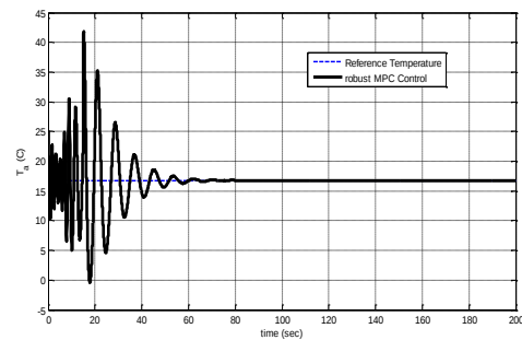
شکل (۱۳): متغیر خروجی دمای هوای داخل اتاق با اعمال کنترل‌کننده‌ی ترکیبی پیش‌بین مقاوم (حالت دوم)
