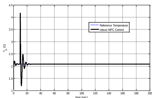
شکل (۱۴): متغیر خروجی دمای سطح تجهیزات دارای اینرسی حرارتی در ساختمان با اعمال کنترل‌کننده‌ی ترکیبی پیش‌بین مقاوم (حالت دوم)
