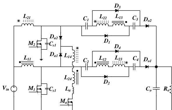
شکل (۱): نمای شماتیک مبدا در هم تنیده بسیار افزاینده پیشنهادی
