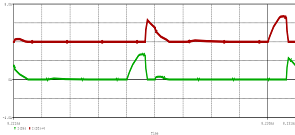
شکل (۱۰): شکل موج جریان دیودهای خروجی D_{a1} و D_{a2} مبدل شبیه سازی شده در مقیاس (1 \mu s/div, 2 A/div)
