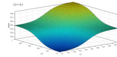
شکل (۴): نمایش سیستم فازی پیشنهادی. الف) نمای سیستم فازی، توابع عضویت ورودی و خروجی (ب)، مشخصه ورودی و خروجی به ازای مقادیر مختلف ورودی L3 (ج).
