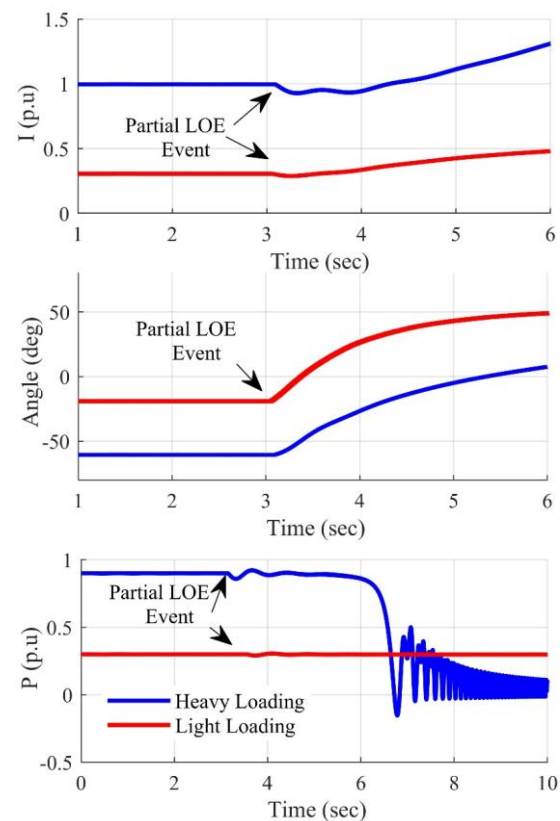
شکل (۹): نتایج شبیه‌سازی وقوع قطع تحریک جزئی تحت بارگذاری مختلف ژنراتور در شرایط بهره‌برداری به صورت فوق‌تحریک.
