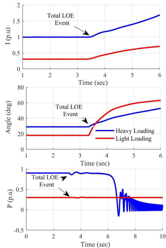
شکل (۴): نتایج شبیه‌سازی وقوع قطع تحریک کامل تحت بارگذاری مختلف ژنراتور در شرایط بهره‌برداری به صورت زیر تحریک.
