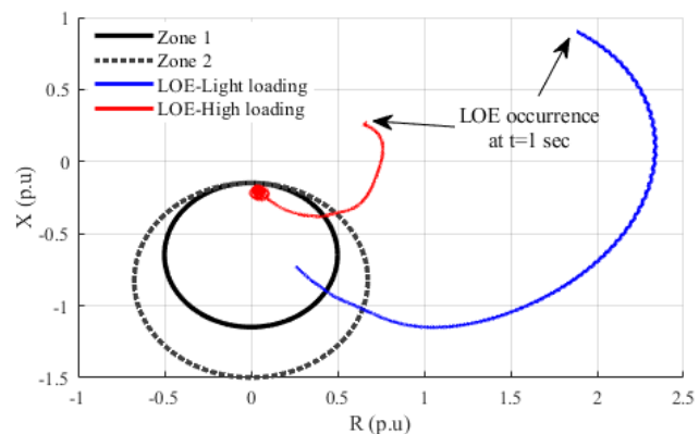
شکل (۱۰): نتایج شبیه‌سازی وقوع قطع تحریک کامل و جزئی تحت بارگذاری سنگین و سبک ژنراتور در شرایط بهره‌برداری به صورت فوق تحریک.
