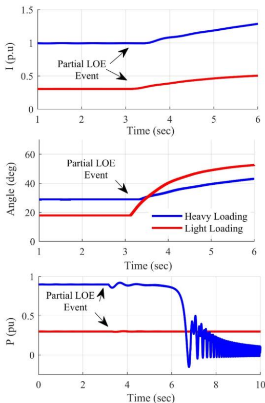
شکل (۶): نتایج شبیه‌سازی وقوع قطع تحریک جزئی تحت بارگذاری مختلف ژنراتور در شرایط بهره‌برداری به صورت زیر تحریک.
