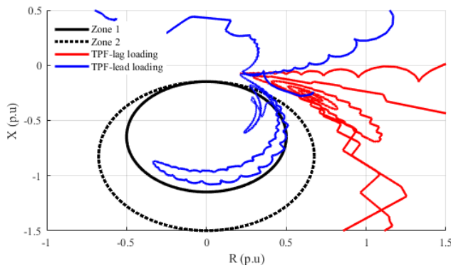
شکل (۱۱): نتایج شبیه‌سازی خطای اتصال کوتاه سه فاز تحت بارگذاری سنگین و سبک ژنراتور در شرایط بهره‌برداری به صورت زیرتحریک.
