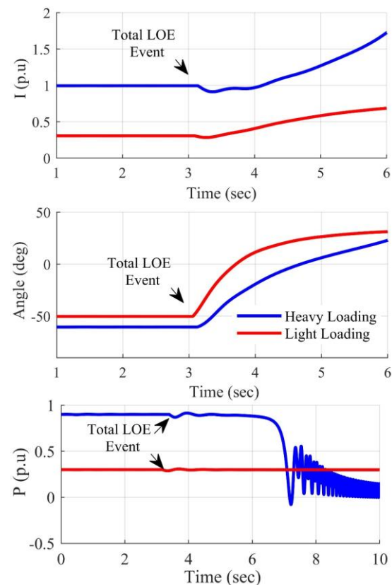
شکل (۵): نتایج شبیه‌سازی وقوع قطع تحریک کامل تحت بارگذاری مختلف ژنراتور در شرایط بهره‌برداری به صورت فوق تحریک.
