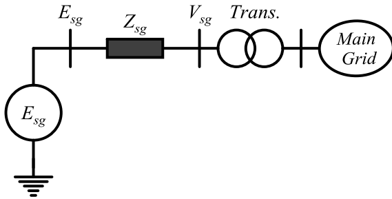
شکل (۲): مدار معادل ژنراتور سنکرون متصل به سیستم قدرت.
