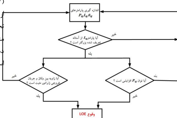
شکل (۳): فلوچارت روش حفاظت قطع تحریک پیشنهادی.
