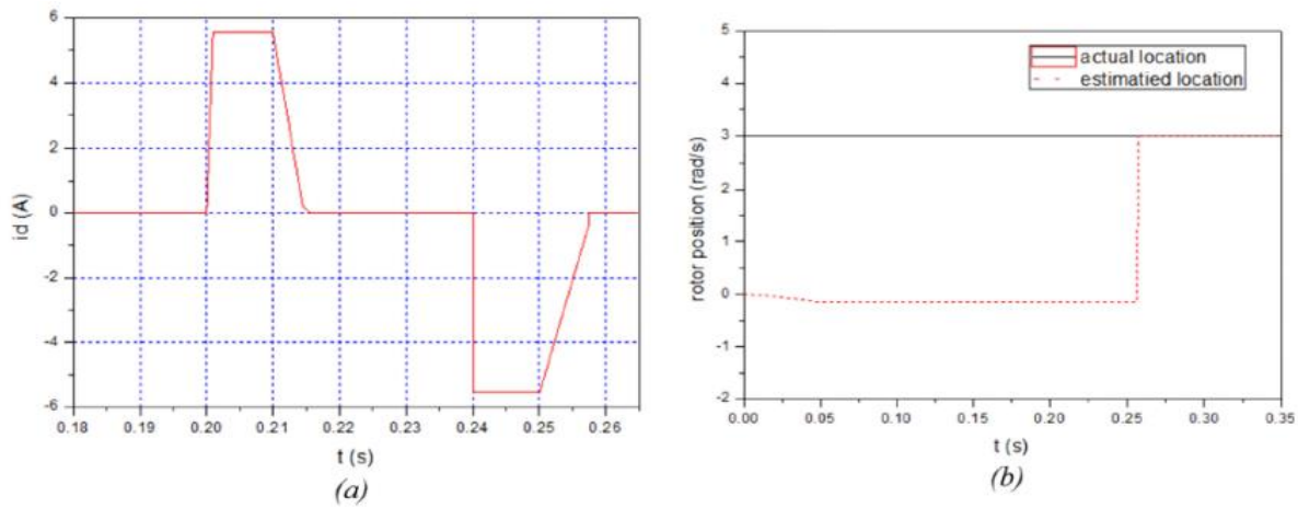
شکل (۱۶): تخمین موقعیت روتور در \theta = 3rad [۹]
