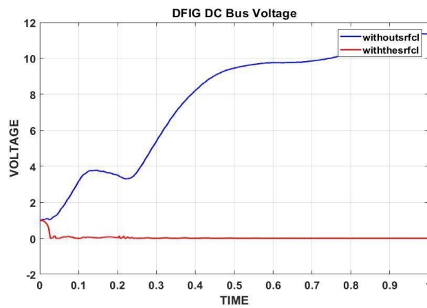
شکل (۲۴)-ولتاژ لینک dc ژنراتور القائی در شرایط باز شدن خط بعد از ژنراتور القائی
