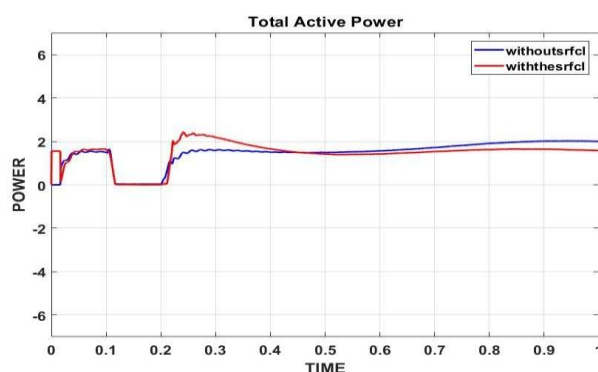
شکل (۲۰)-توان کل شبکه تحت خطای سه فاز قبل از ژنراتور القائی
