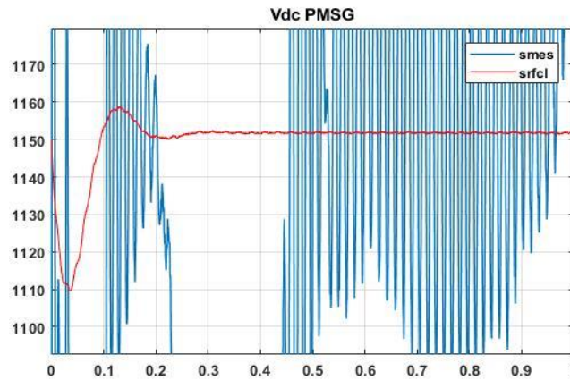
شکل (۲۳)-ولتاژ لینک dc ژنراتور سنکرون مغناطیس دائم در شرایط باز شدن خط بعد از ژنراتور القائی
