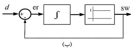
شکل (۲): (الف) استراتژی کنترل پیشنهادی و (ب) مدولاتور دلتاسیگما تک‌بیتی.
