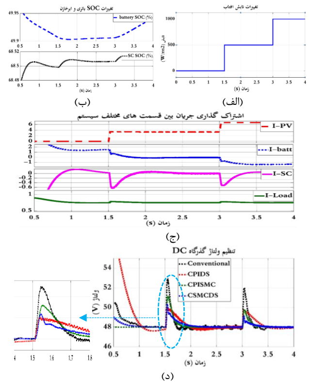
شکل (۵): نتایج سناریوی دوم الف: تابش؛ ب: SOC باتری و ابرخازن؛ ج: جریان بخش‌های مختلف؛ د: مقایسه گذرگاه DC
