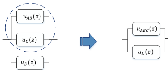
شکل (۶): ترکیب موازی تابع u_C(z) و u_{AB}(z) Figure (6): Parallel function composition u_{AB}(z) , u_C(z)
