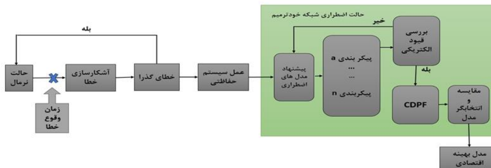
شکل (۱): مدل پیشنهادی برای بازیابی خودترمیم (حالت اضطراری) تحت شرایط شکست سخت
