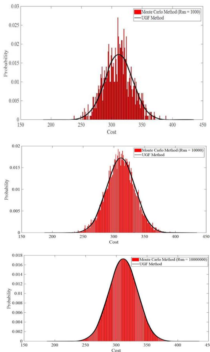
شکل (۱۲): مقایسه دقت روش UGF و مونت کارلو با الف) هزار تکرار ب) ده هزار تکرار ج) ده میلیون تکرار
