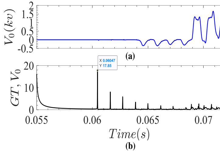
شکل (۱۳): (a) مؤلفه توالی صفر ولتاژ (V_0) ، (b) سیگنال گابور متناظر با V_0 -سناریوی ۳
