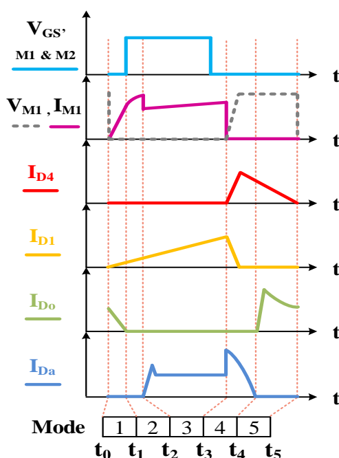
شکل (۳): شکل موجهای کلیدی مبدل افزایشنده پیشنهادی Figure (3): Key waveforms of the proposed step-up converter
