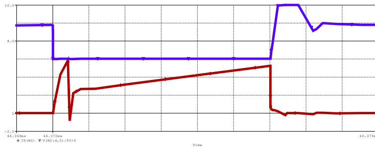
شکل (۸): شکل موج های شبیه سازی ولتاژ درین- سورس (بالا) و جریان (پایین) سوئیچ M_2 (2A/div, 50V/div, 1 \mu s/div) Figure (8): Simulation waveforms of drain-source voltage (top) and current (bottom) of switch M_2 (2A/div, 50V/div, 1 \mu s/div)
