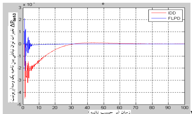
ج: تغییرات توان تبادل بین ناحیه ۱ و ۳
