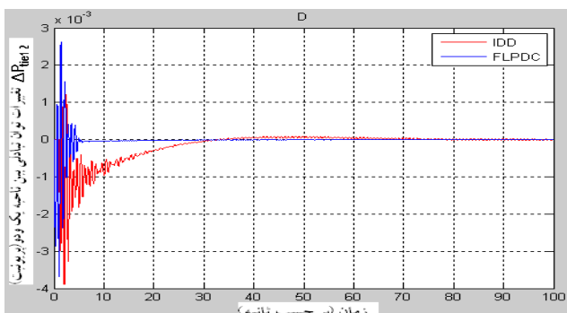
ت: تغییرات توان تبادل بین نواحی ۱ و ۲
