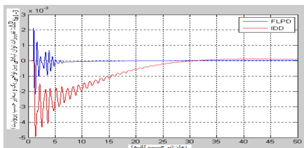
ت: تغییرات توان تبدیلی بین نواحی ۱ و ۳
