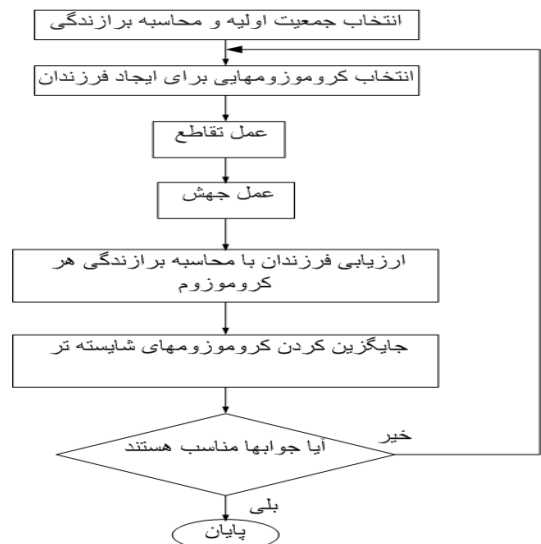
شکل (۴): فلوچارت مراحل اجرای الگوریتم ژنتیک
