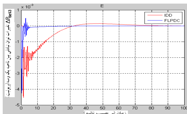
ش: تغییرات توان تبدیلی بین نواحی ۱ و ۳ شکل (۷): مقایسه عملکرد کنترلر فازی و کنترلر IDD بعد از تغییر پارامترهای سیستم قدرت
