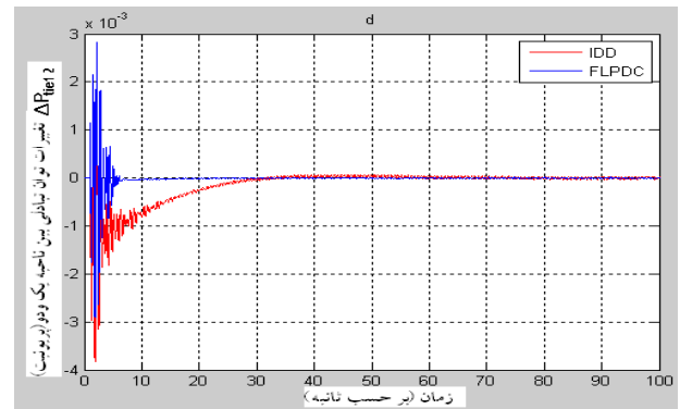
ث: تغییرات توان تبادل بین ناحیه ۱ و ۲
