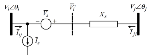
شکل ۲- مدار معادل عنصر UPFC
