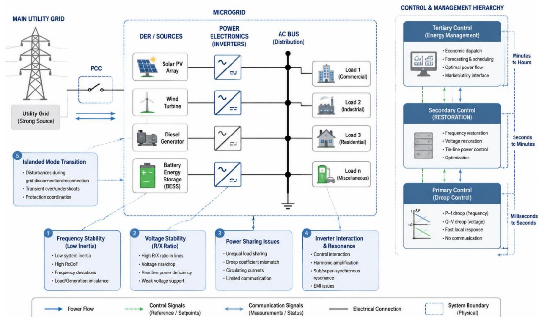
شکل (۸): ساختار نمونه یک ریزشکه برای بررسی چالش‌های پایداری در حالت‌های متصل به شبکه و جزیره‌ای Figure (8-2): Sample structure of a microgrid to investigate stability challenges in grid-connected and islanded modes
