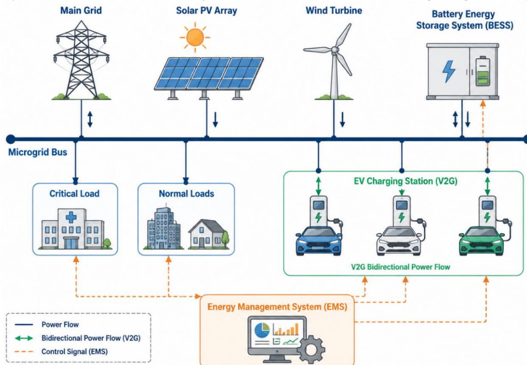
شکل (۴): شماتیک یک ریزشکبه مجهز به فناوری خودرو به شبکه
