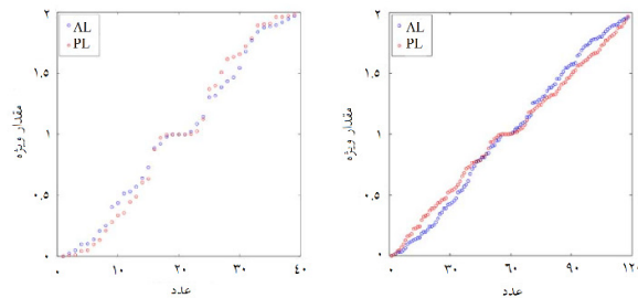
شکل ۸ مقادیر ویژه برای توان عبوری مبتنی بر (PL) و ادمیتانس مبتنی بر (AL) لاپلاسن نرمالیزه شده سیستم آزمایشی ۳۹ شینه IEEE (چپ)، سیستم آزمایشی ۱۱۸ شینه IEEE (راست).
