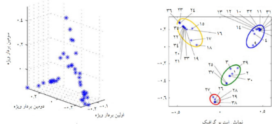
شکل ۵ جایگیری طیفی با ابعاد ۳ برای نمونه آزمایشی ۳۹ شینه IEEE، توان عبوری (چپ) و نمایش استریوگرافیک (راست).
